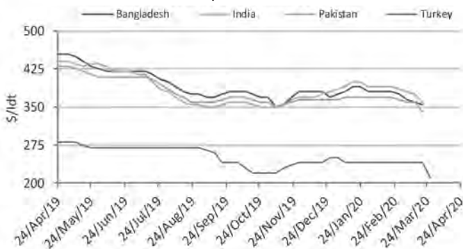
Цены на танкеры 24.04.19-24.04.20
