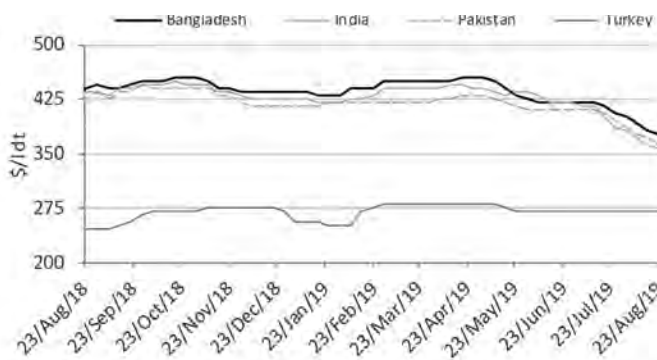
Цены на танкеры 23.08.18-23.08.19
